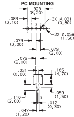
OS102011MS2QN1 SPDT
