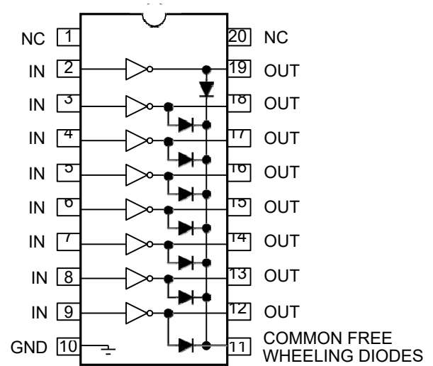
SOP-20/TSSOP-20
