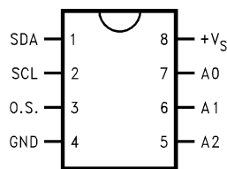
SOP-8 and Mini SOP-8
