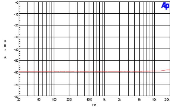
17. CMRR
