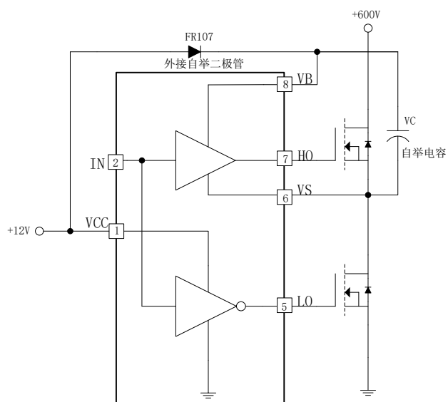
图 8-3. EG2104M 自举电路结构
