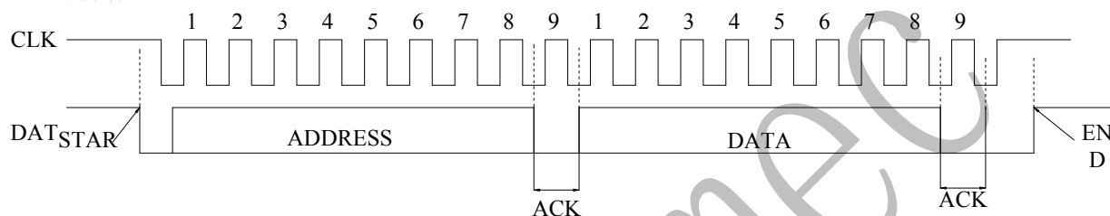
图 3 写显示时序
