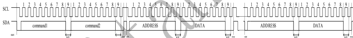
图 4 完整时序
