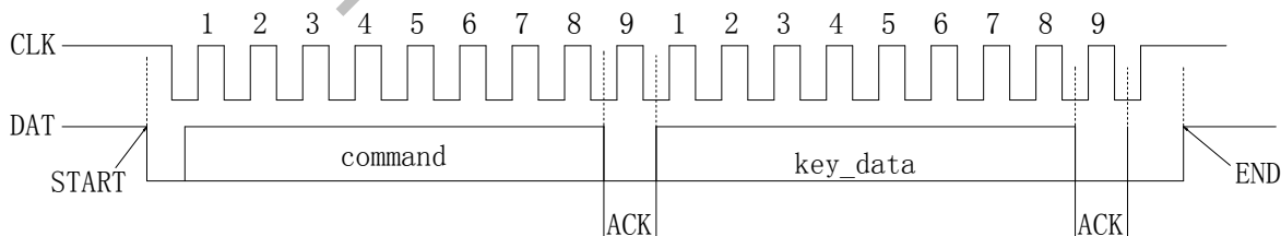
图 5 读按键时序
