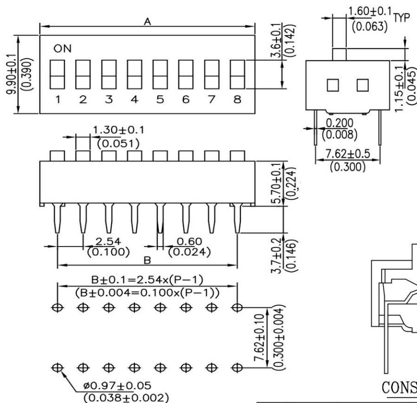
P.C.B. LAYOUT
