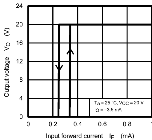
Fig. 12.2.4 V_O - I_F(I_{HYS})
