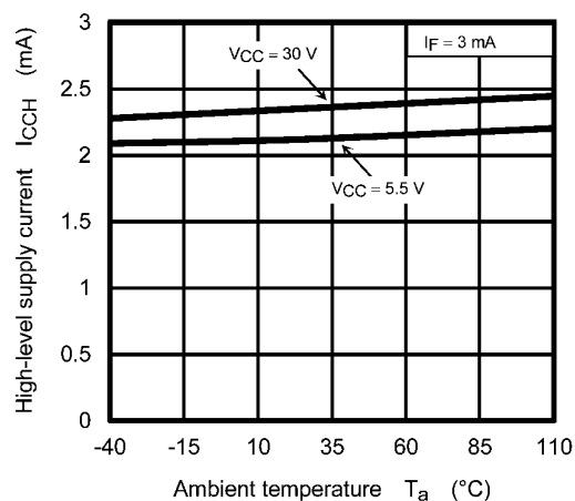
Fig. 12.2.8 I_{cCH} - T_a
