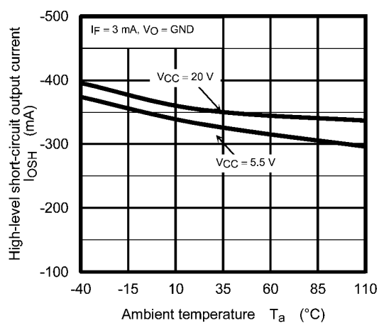
Fig. 12.2.10 I_{osH} - T_a
