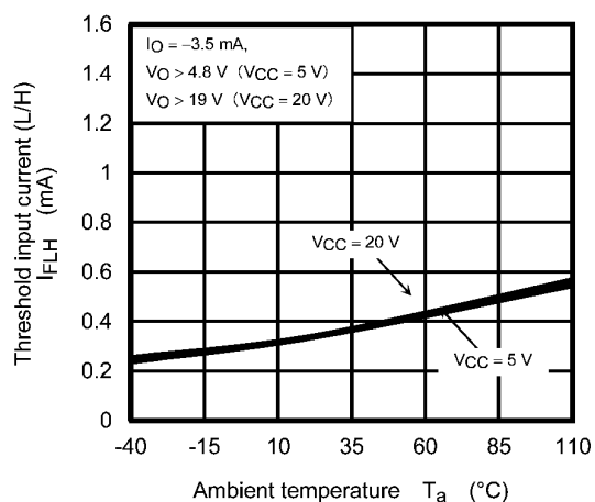
Fig. 12.2.2 I_{FLH} - T_a
