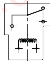
转换 C 型
