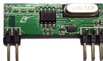
RFM210LCF-A
