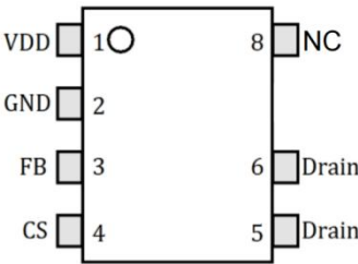
SOP-7俯视图
