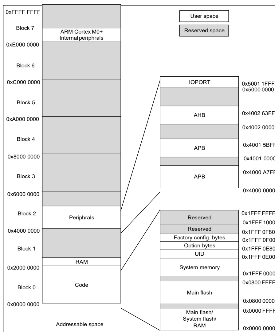
图 5-1 存储器映射
