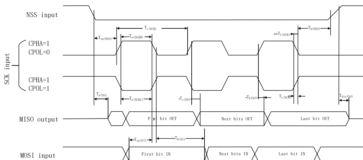
图 6-3 SPI 时序图-slave mode and CPHA=1
