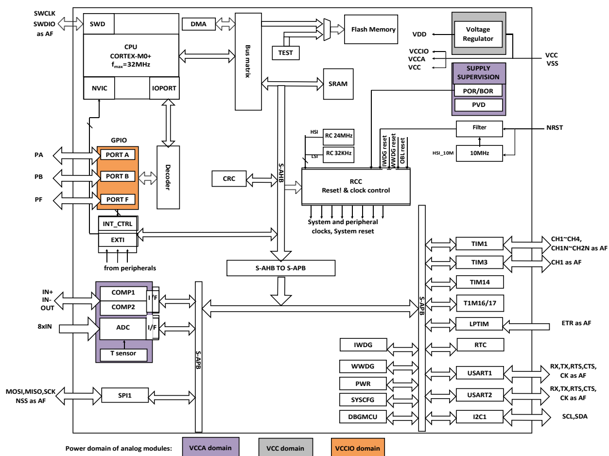
图 2-1 功能模块
