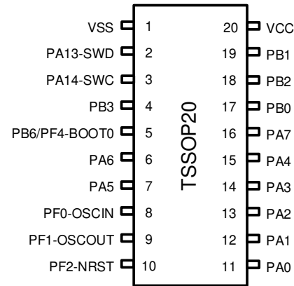
图 3-4 TSSOP20 Pinout1 PY32F002AF15P
