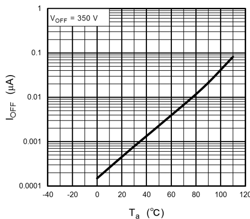
Fig. 14.1.9 I_{OFF} - T_a
