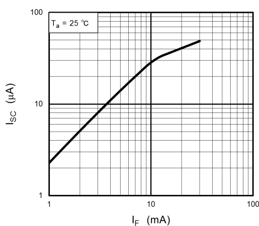
Fig. 12.5 I_{SC} - I_F
