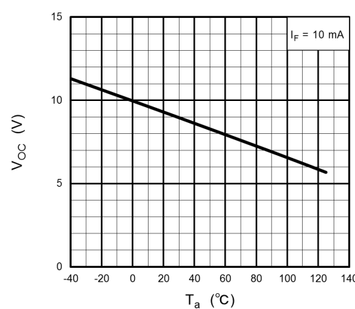
Fig. 12.6 V_{OC} - T_a
