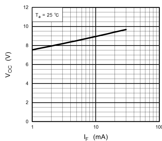
Fig. 12.4 V_{OC} - I_F
