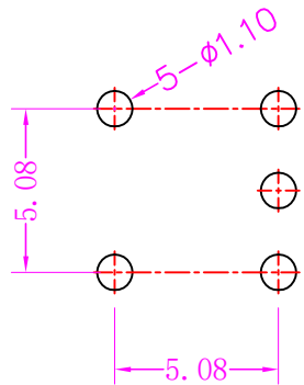
安装孔尺寸
