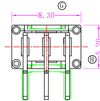
手柄位置及导通端子示意图
