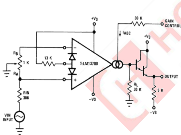
图 12 电压控制放大器
