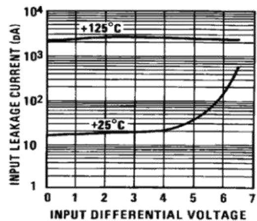
图 6 输入漏电流
