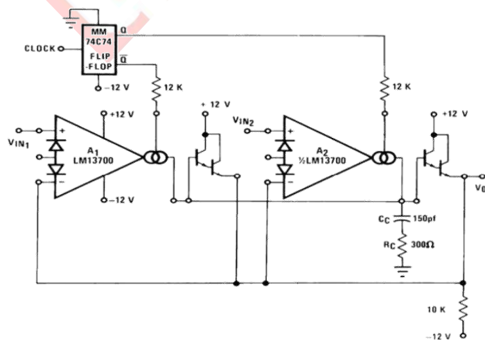
图 19 多路复用器
