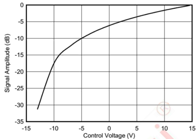
图 11 信号幅度与控制电压
