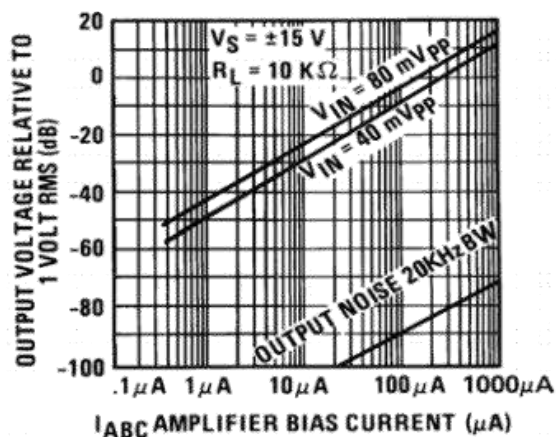
图 8 输出电压与运放偏置电流
