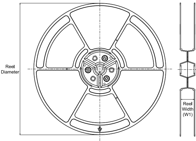
REEL DIMENSIONS
