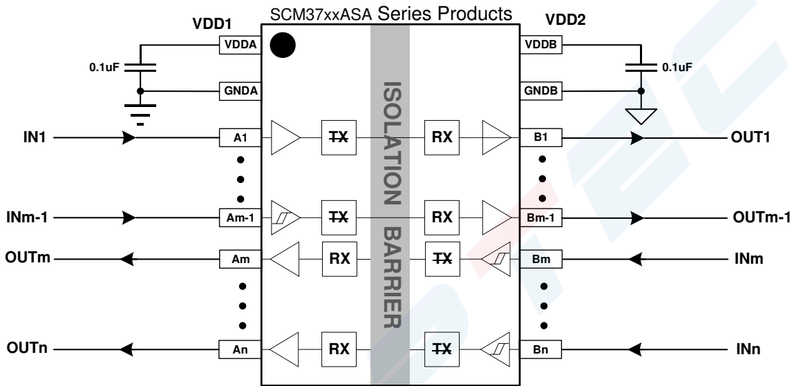
图10-1 SCM37xxASA 系列数字隔离器应用原理图
