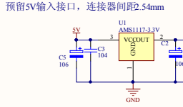
供电稳压供电
