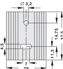
SK 09 37,5 TO 220
