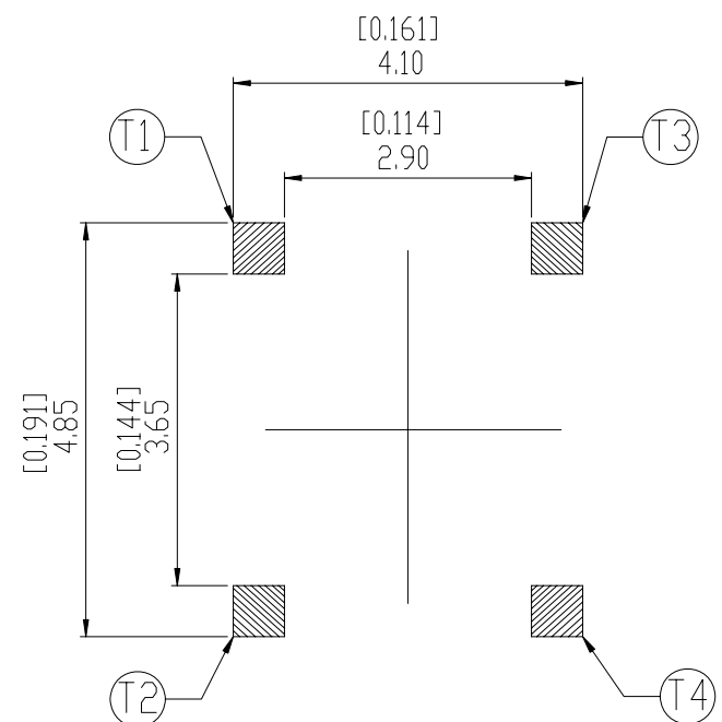
P.C.B. LAYOUT
