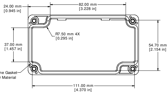
LID - INSIDE
